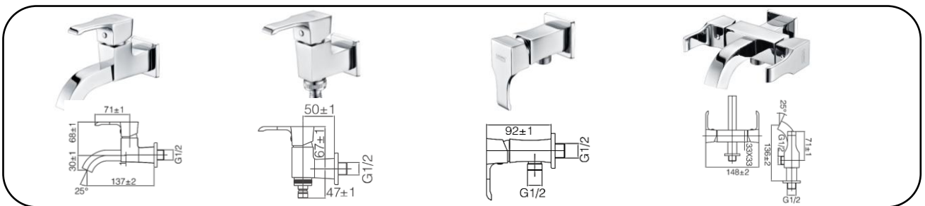
VT5905 Bib tap
